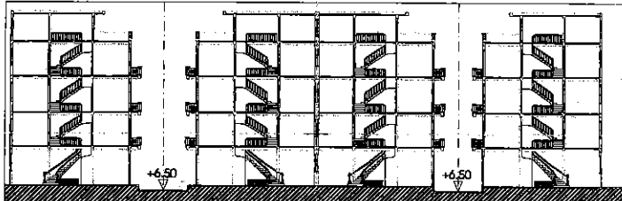
MẶT CẮT KHAI TRIỂN 1 - 1
